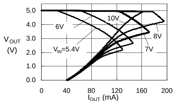
S-817A50A (Ta=25°C)
