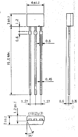
図3 SPT
