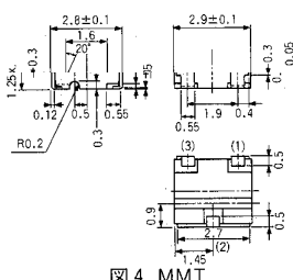
図4 MMT
