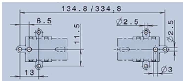
Montagebohrungen · Mounting holes
