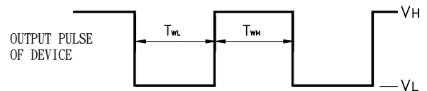
D.U.T output Pulse
