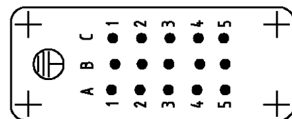
Kontaktanordnung Contact arrangement
