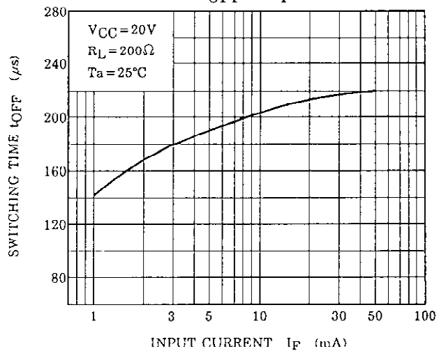
t_{OFF} - I_F
