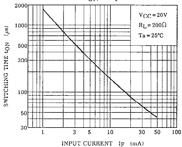
t_{ON} - I_F
