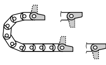
10...2P(Z) Festpunkt mit Bolzen (Innenlasche)
