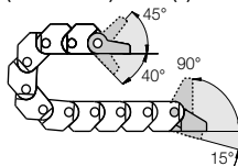
11...2P(Z) Festpunkt mit Bolzen (Innenlasche)
