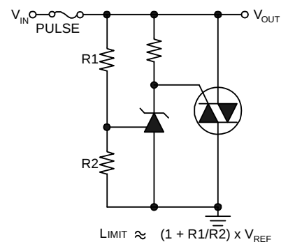
Fig. 9 Crow Bar
