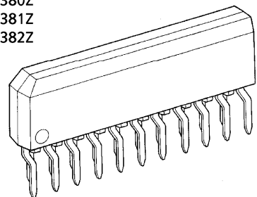
SZIP21-P-0.89
