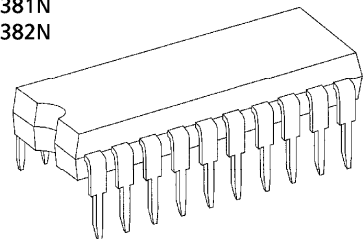
SDIP20-P-300-1.78
