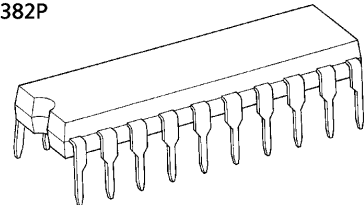
DIP20-P-300-2.54A
