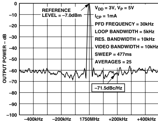
TPC 8. ADF4118 Phase Noise (1750 MHz, 30 kHz, 3 kHz)
