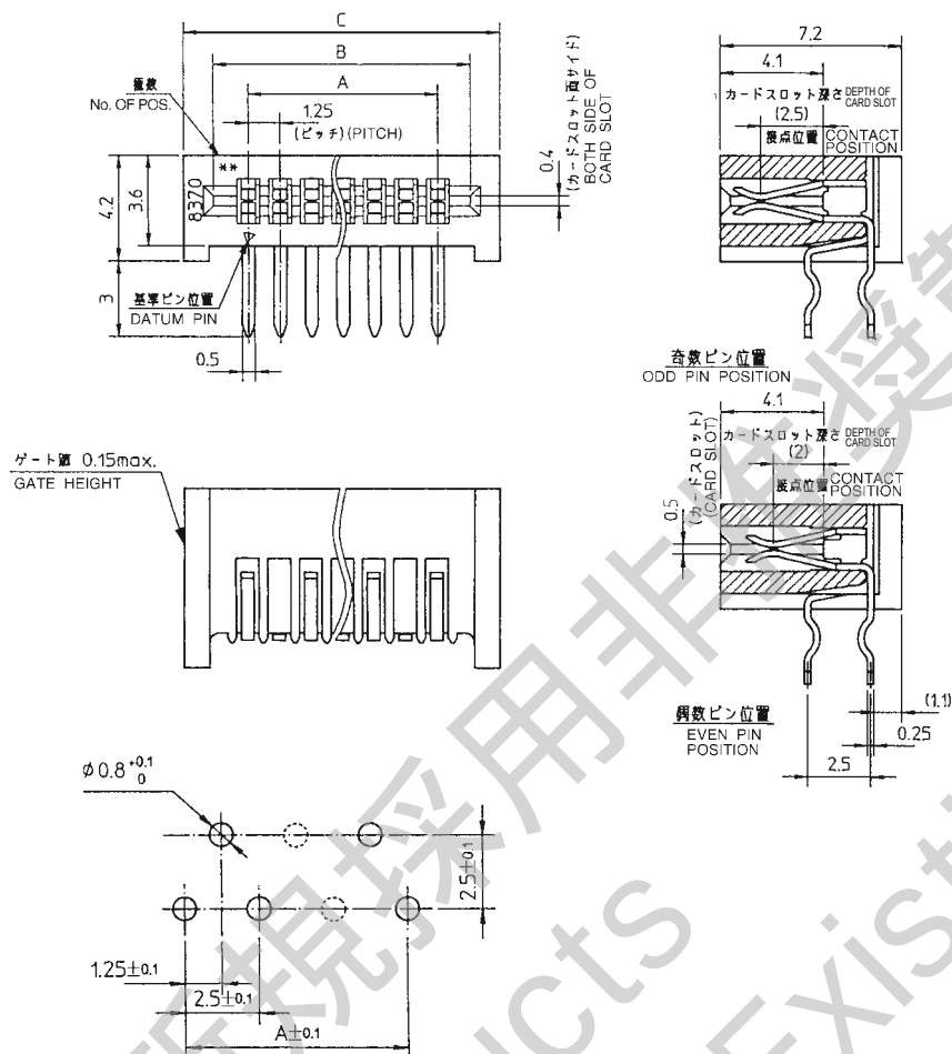
基板穴明寸法 (コネクタ搭載面) MOUNTING LAYOUT
