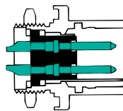
Receptacle «D»
