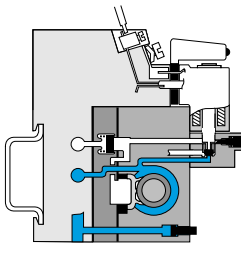
4/2 bistable module
