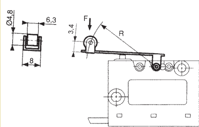
161E roller
