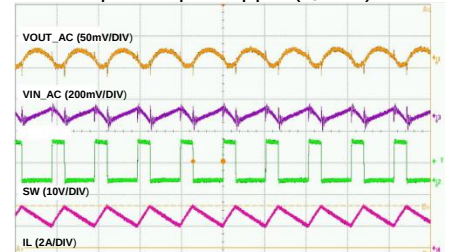
Input/Output Ripple (I O =2A)
