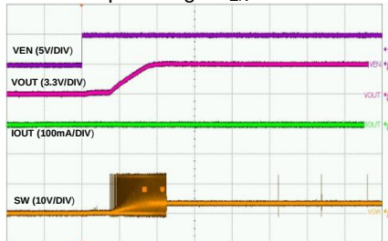
Startup Through V EN 0A Load
