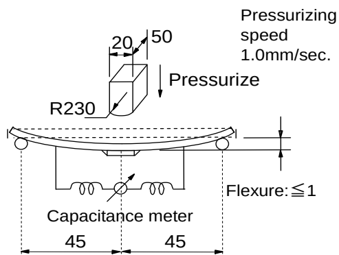
Fig.2 (in:mm)
