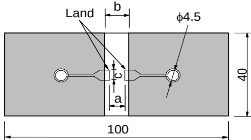
Fig.1 (in:mm)
