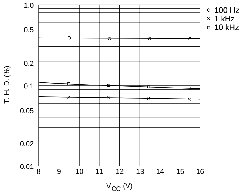
HA12142NT
