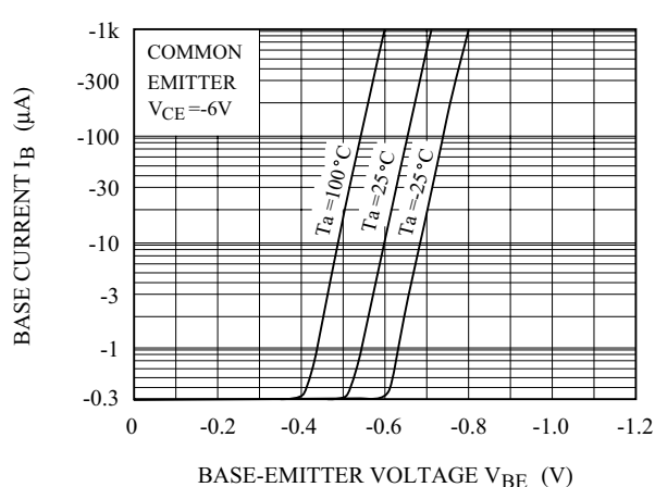
I_B - V_{BE}
