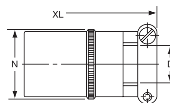
MS3116J-XX-XXX
