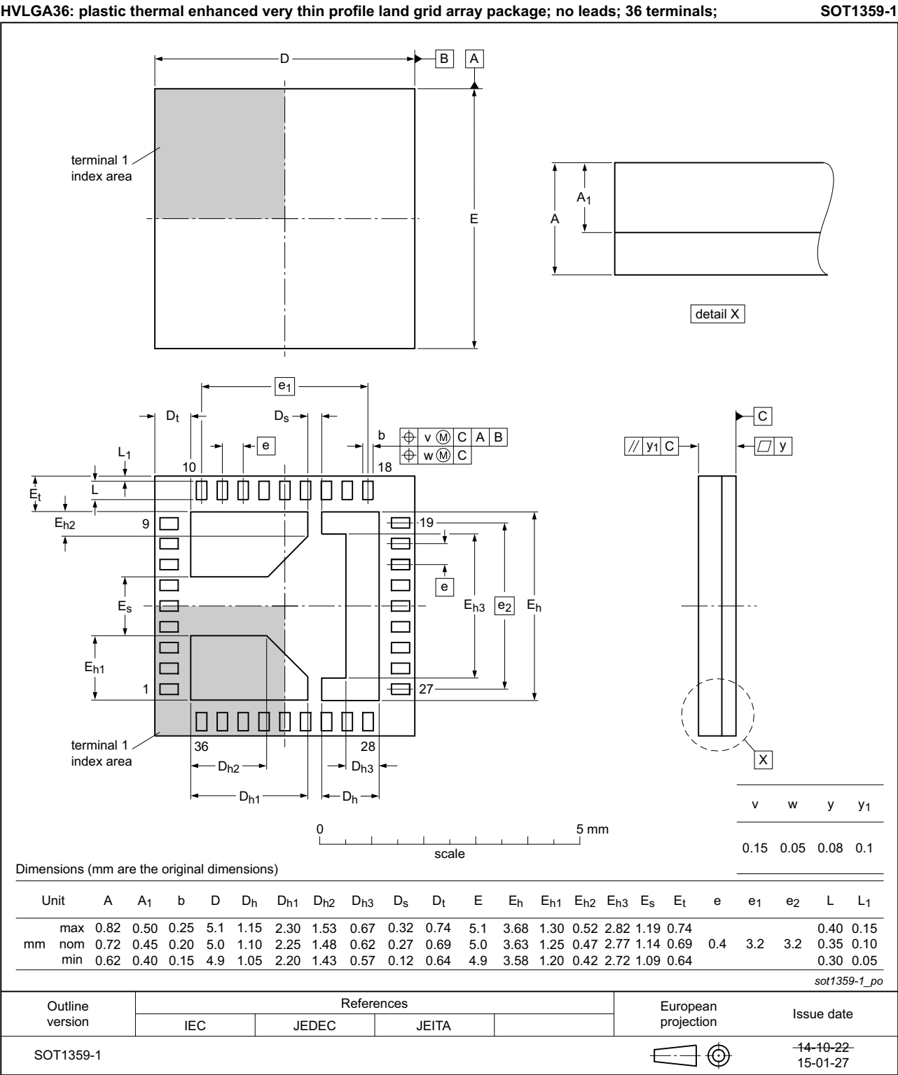
Fig 30. Package outline SOT1359-1 (HVLGA36)
