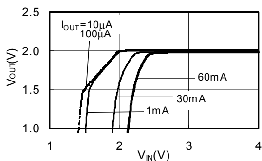
S-818A20A ( T_a=25^\circ\text{C} )
