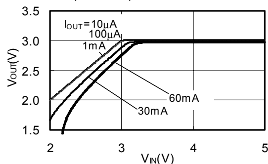
S-818A30A ( T_a=25^\circ\text{C} )
