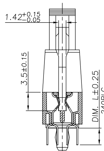
SECT B-B SCALE 2:1
