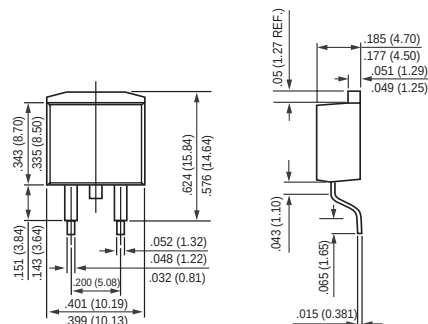
D2PAK
