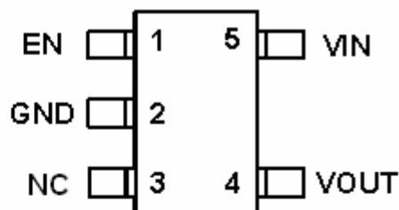
SOT-23-5B / SC-70B
