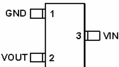
SOT-23-3A
