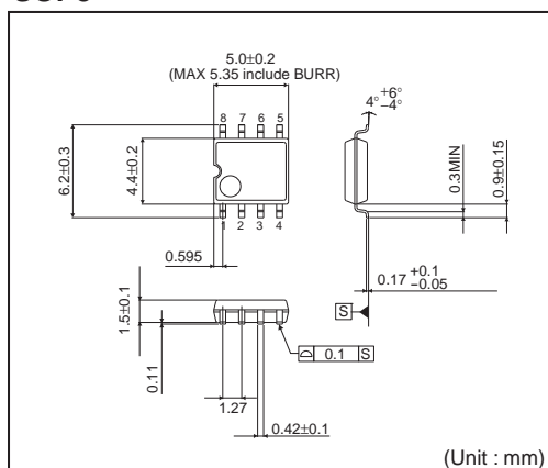
(Unit : mm)
