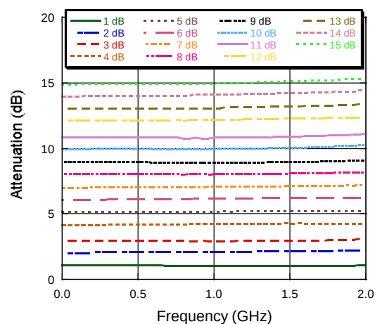
Attenuation
