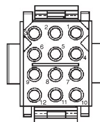
Receptacle
