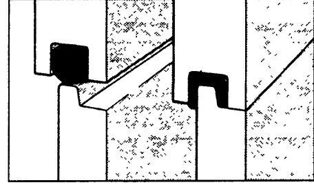
Deckeldichtung im Feder-Nut-System Lid seal in tongue and groove system
