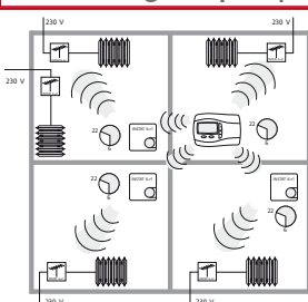
Zeitsteuerung mit Master und Slaveregler Time control with master and slave units
