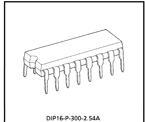
DIP16-P-300-2.54A Weight : 1.00g (Typ.)
