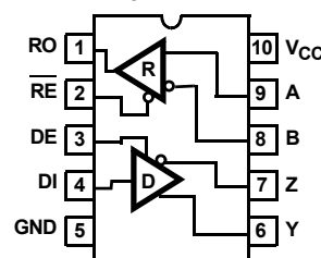
ISL32600E, ISL32602E (10 LD MSOP)
