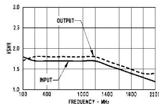
VSWR
