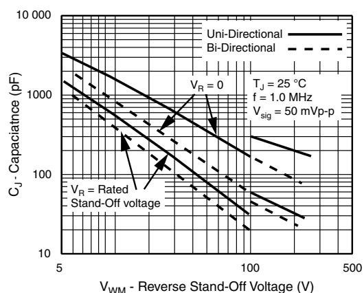
Fig. 6 - Capacitance
