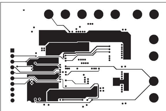
Copper Layer 3
