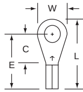
L-11-8 Stud Size 8 Wire Range 22-18
