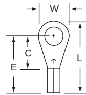
L-11-10 Stud Size 10 Wire Range 22-18
