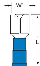
72F-250-32-NB Wire Range 16-14
