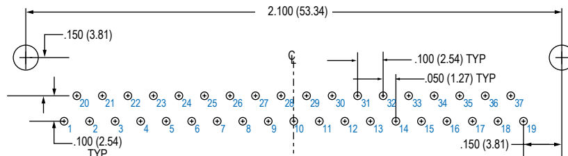
37 SOCKET
