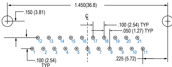
21 SOCKET
