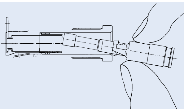
c) Beim Einsetzen oder Auswechseln eines G-Sicherungseinsatzes können weder über den Sicherungseinsatz, noch den Sicherungseinsatzträger aktive Teile berührt werden.
