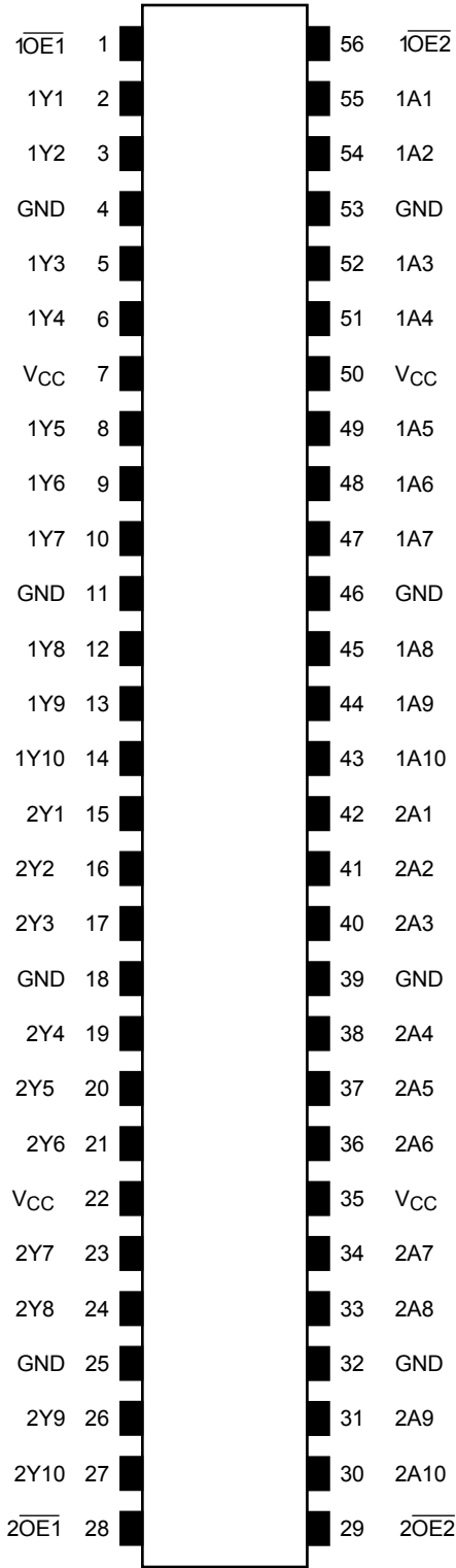
ピン接続図 (top view)
