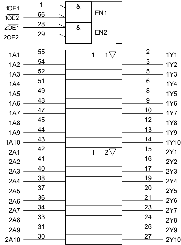
論理図
