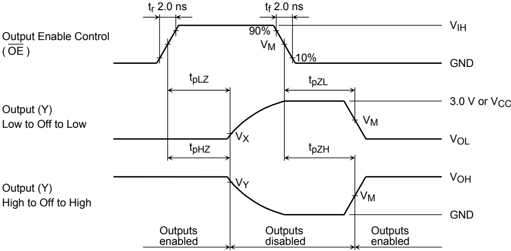
図 3 t_{pLZ} , t_{pHZ} , t_{pZL} , t_{pZH}
