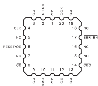
20-pin PLCC
