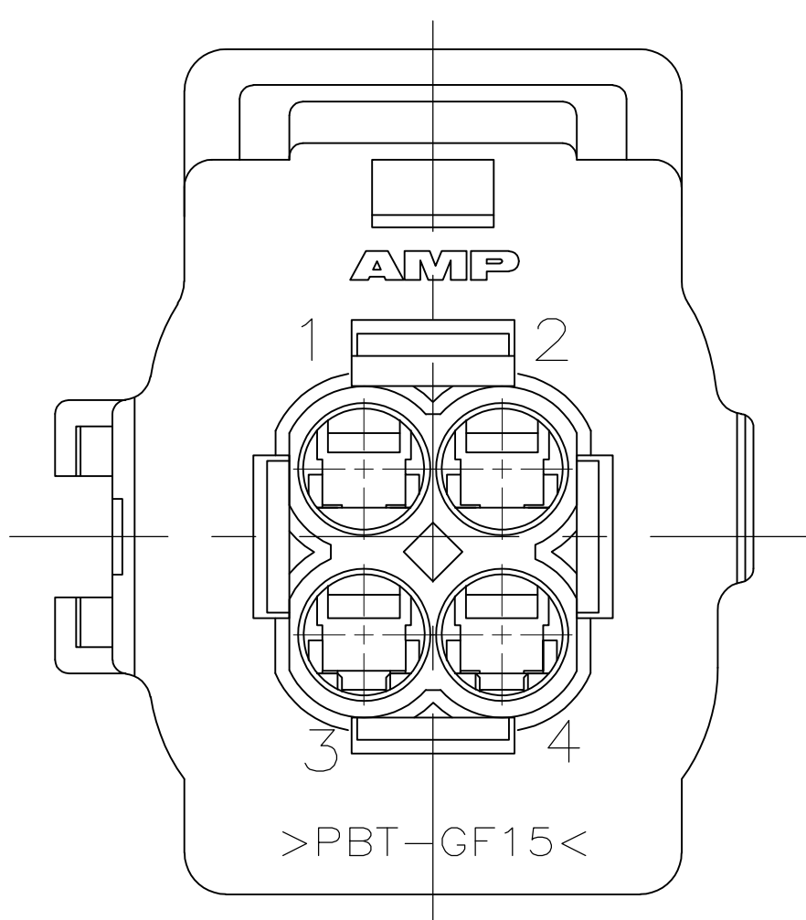
VIEW A-A
