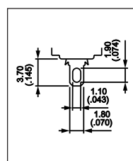
Solder lug
