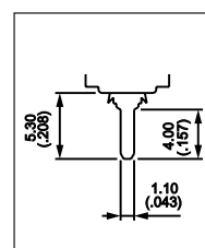
Straight p.c.
