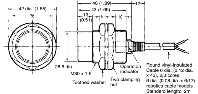
Fig. 8: E2E-X18MY□-N
