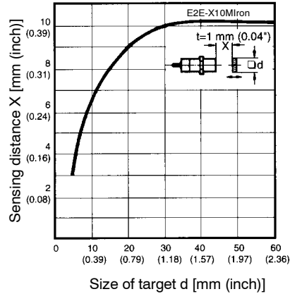
E2E-X10M□□
