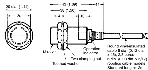
Fig. 5: E2E-X5Y□-N
