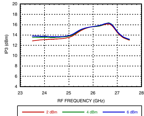
Input IP3, USB vs. LO Drive
