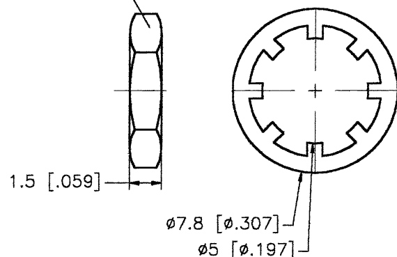
6 HEX NUT
