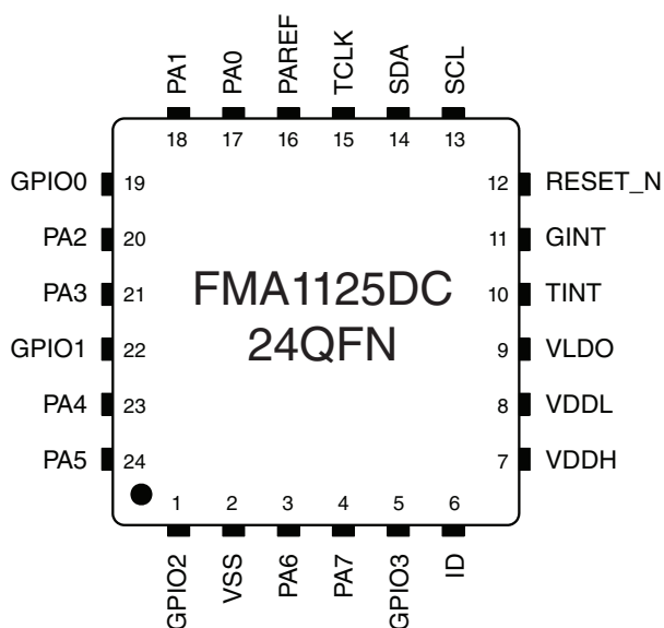
24-Pin QFN
