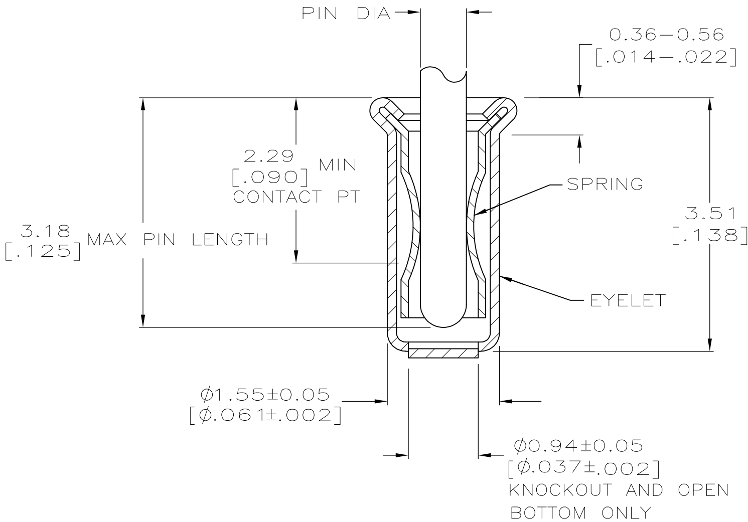
SECTION A-A
