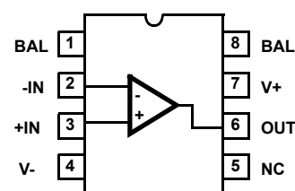
HA-5147 (CERDIP)
