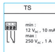
Wiring schematic
