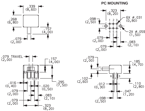
Actuator shown in pos. 1
