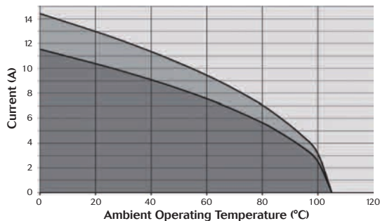
UTS Hi seal 10E6 10D6
