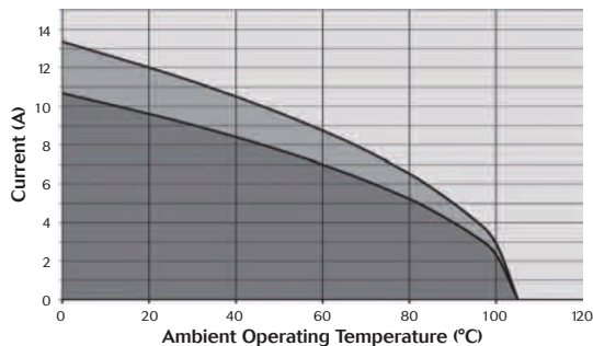
UTS Hi seal 10E7 10D7
